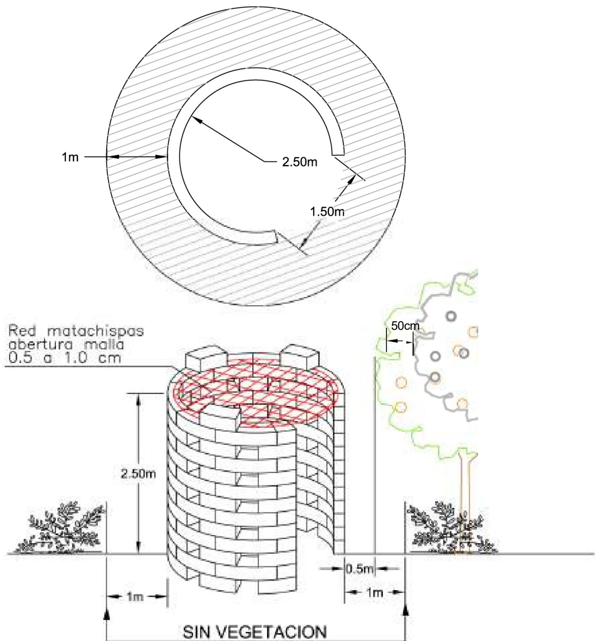
Figura 1. Plantayaizado de un quemador debidamente acondicionado.
